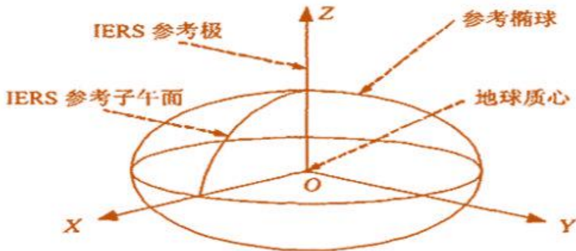
CGCS2000 定义的示意图
